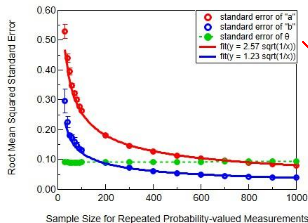
離散データ行列(n=50)+ 確率データ行列(このサンプルサイズを 様々変動させる)を一体的に分析
