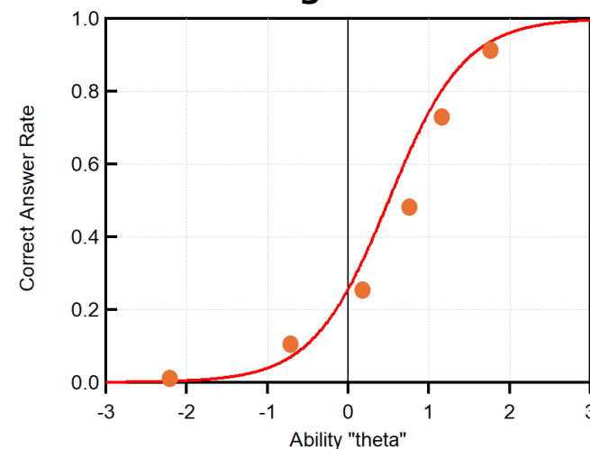
fittingのイメージ
